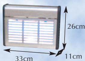
ATRIUM 30 G i/L
